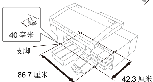
抗震固定示例
