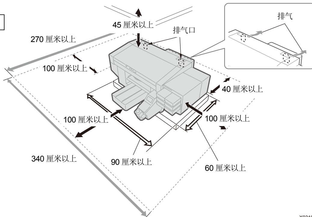
打印机设置尺寸
