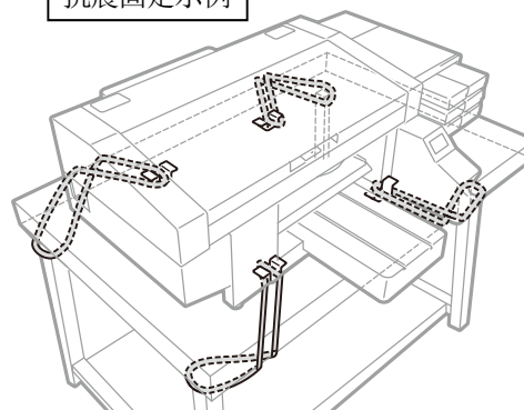
抗震固定示例
